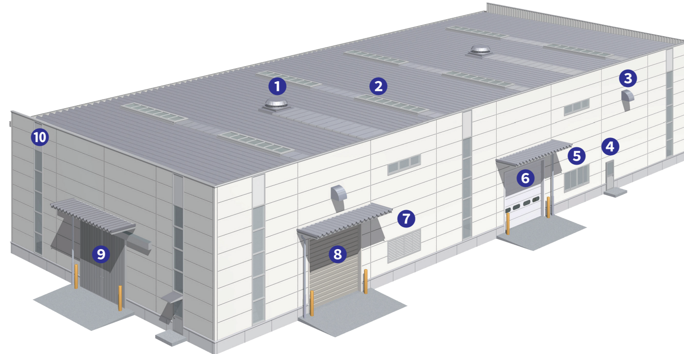
⑥ SP オーバードア 外壁システム対応の標準オーバードア
