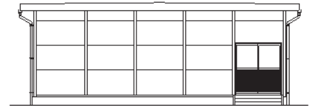
立面図 S1/100
