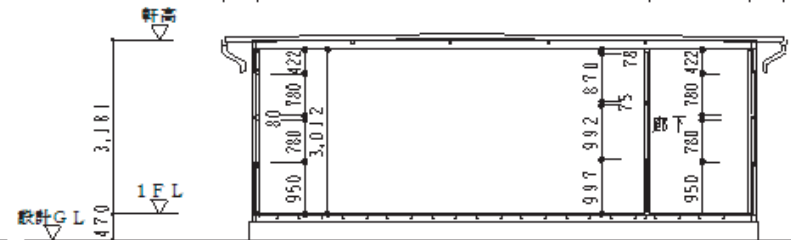
断面図 S1/100
