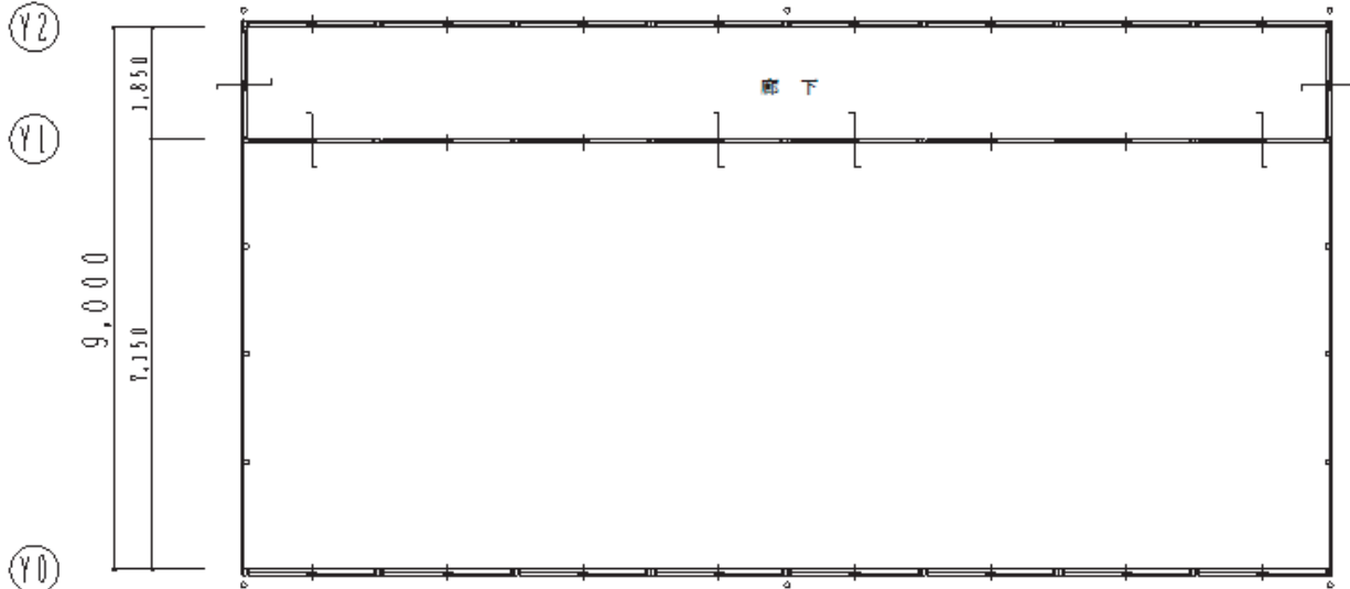
平面図 S1/100
