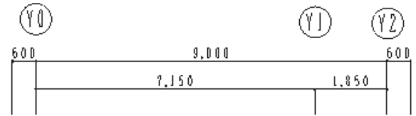
立面図 S1/100
